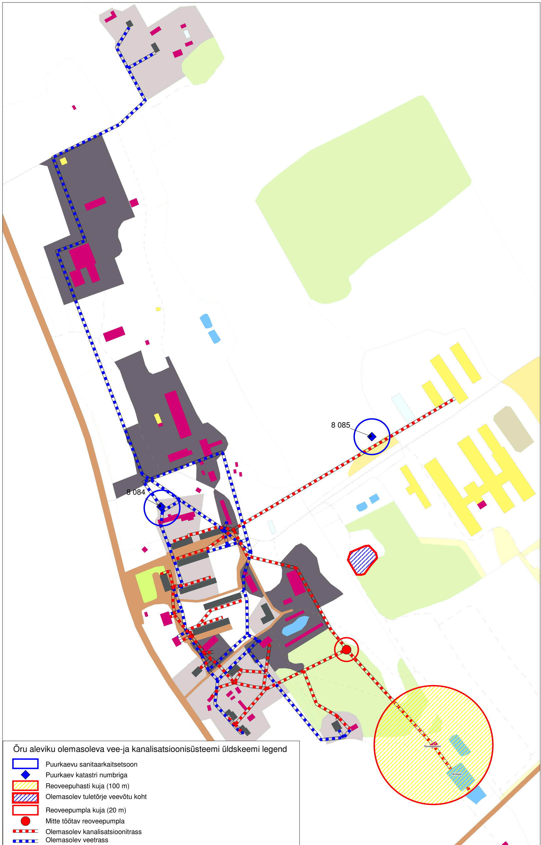
Lisa 1a: Öru aleviku olemasolev ühisveevarustuse ja kanalisatsiooni üldskeem
