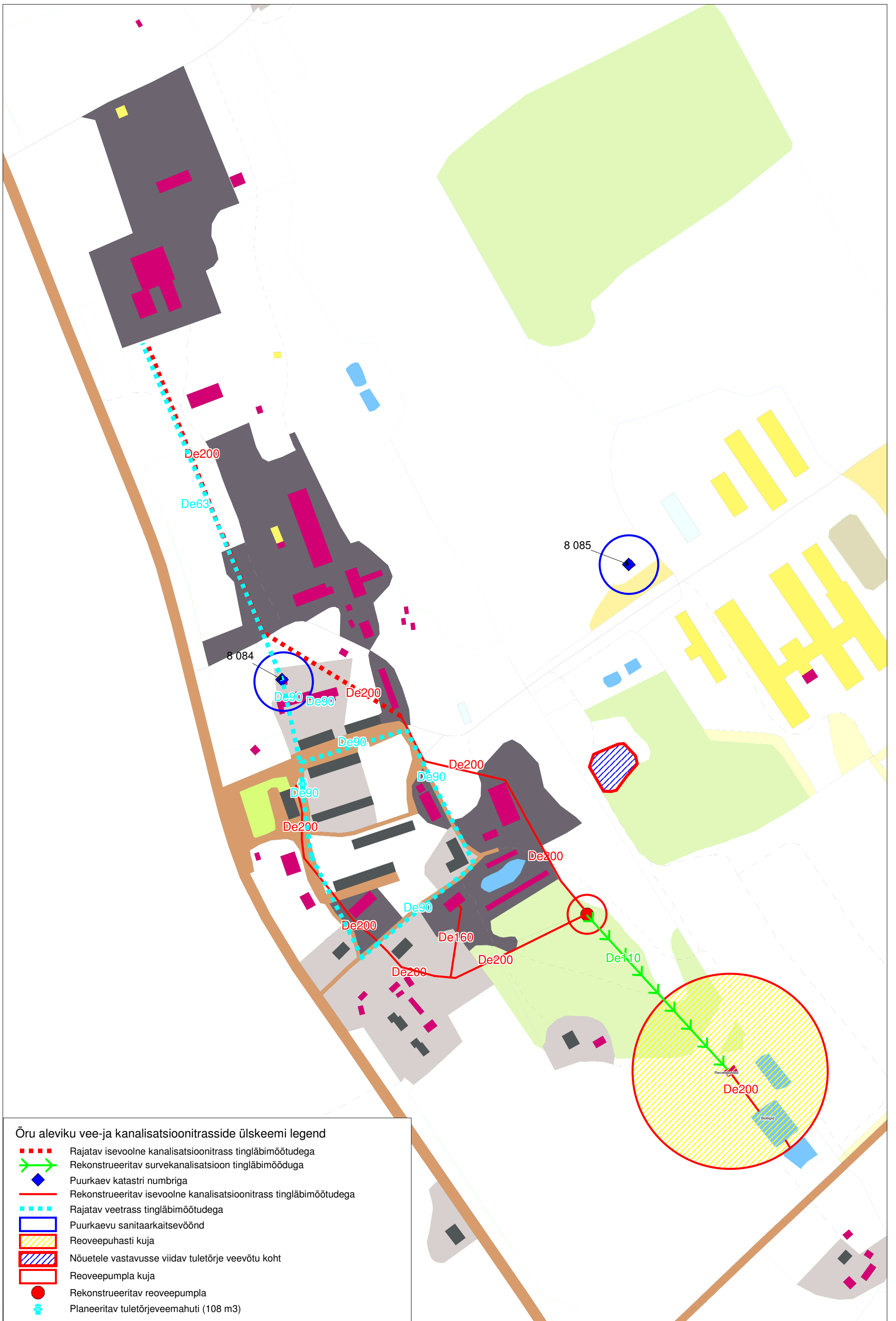
Lisa 1b: Öru aleviku rekonstrueeritava ja rajatava ühisveevarustuse-ja kanalisatsiooni üldskeem
